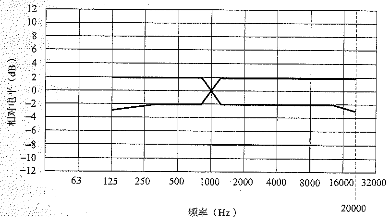
图 3.2.1-3 高品质数字红外线同声传译系统的传输频率响应的允许范围
